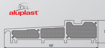
Próg 279110
