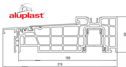
Próg Thermostep 204
