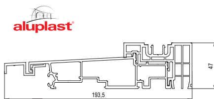
Próg GU-47
