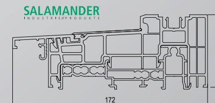
Próg Thermostep
